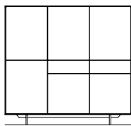
NYR VIT LAAG NR. 338 B 1682 mm / H 1570 mm / D 475 mm
