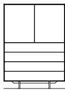
NYR VIT LAAG NR. 313 B 1128 mm / H 1570 mm / D 475 mm
