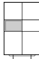
NYR VIT HOOG NR. 422 B 1128 mm / H 1747 mm / D 475 mm
