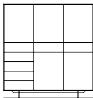
NYR VIT HOOG NR. 431 B 1682 mm / H 1747 mm / D 475 mm
