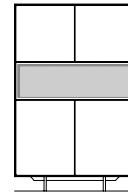
NYR VIT HOOG NR. 414 B 1128 mm / H 1747 mm / D 475 mm
